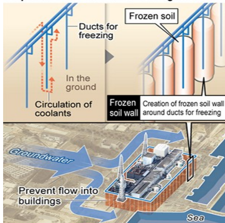
Fal talajfagyasztással
